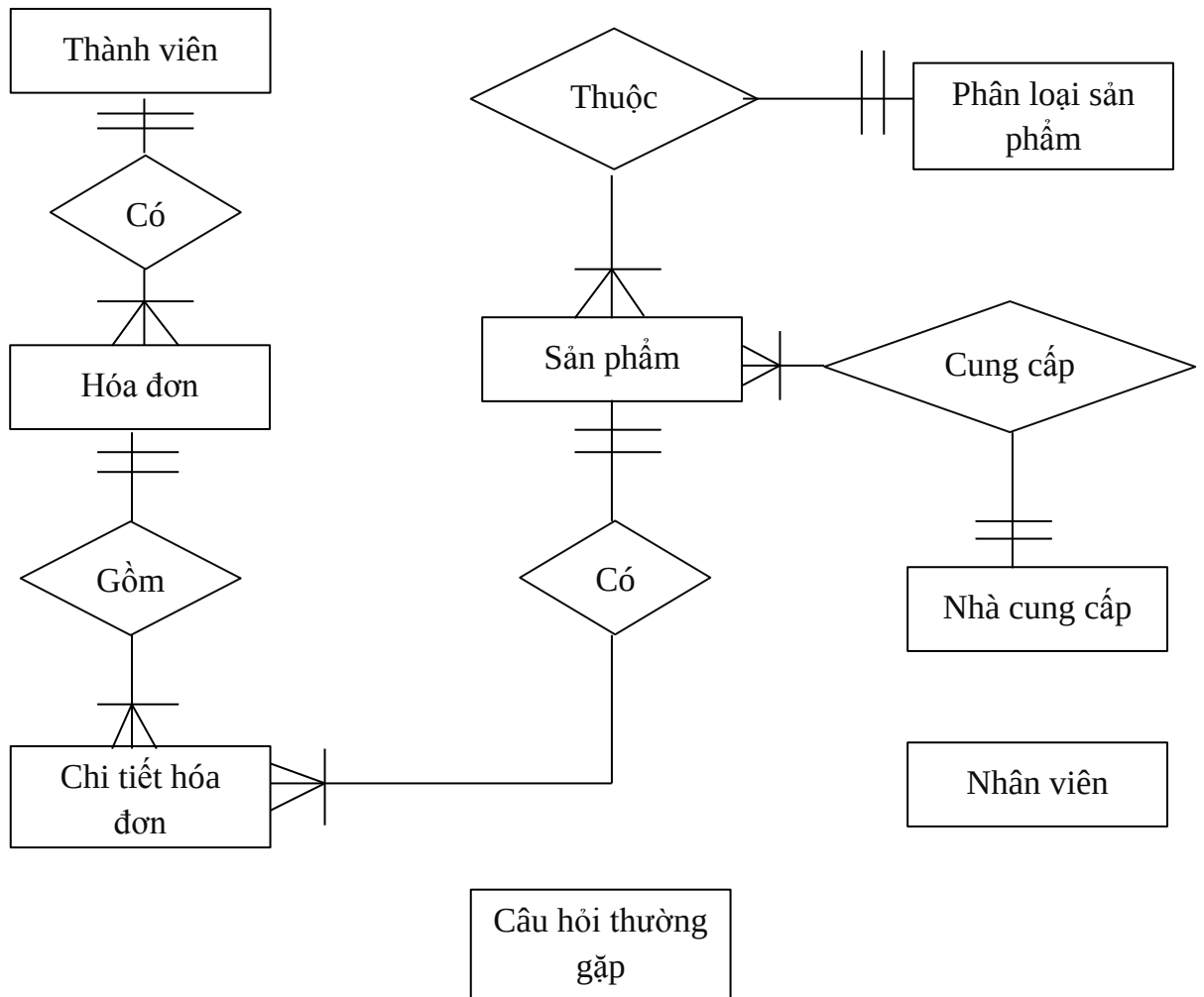
Hình 9: Biểu đồ ERD
