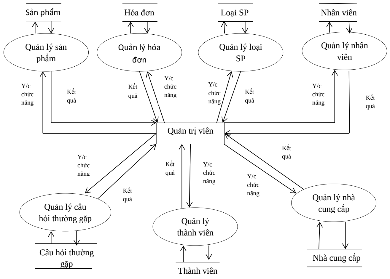
Hình 8: Mức 1- Tiến trình quản trị
