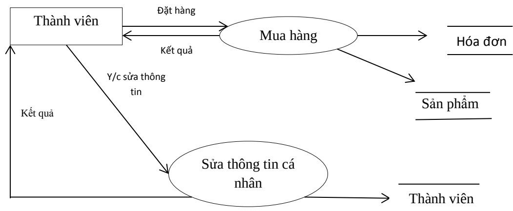
Hình 6: Mức 1- Tiến trình thành viên
