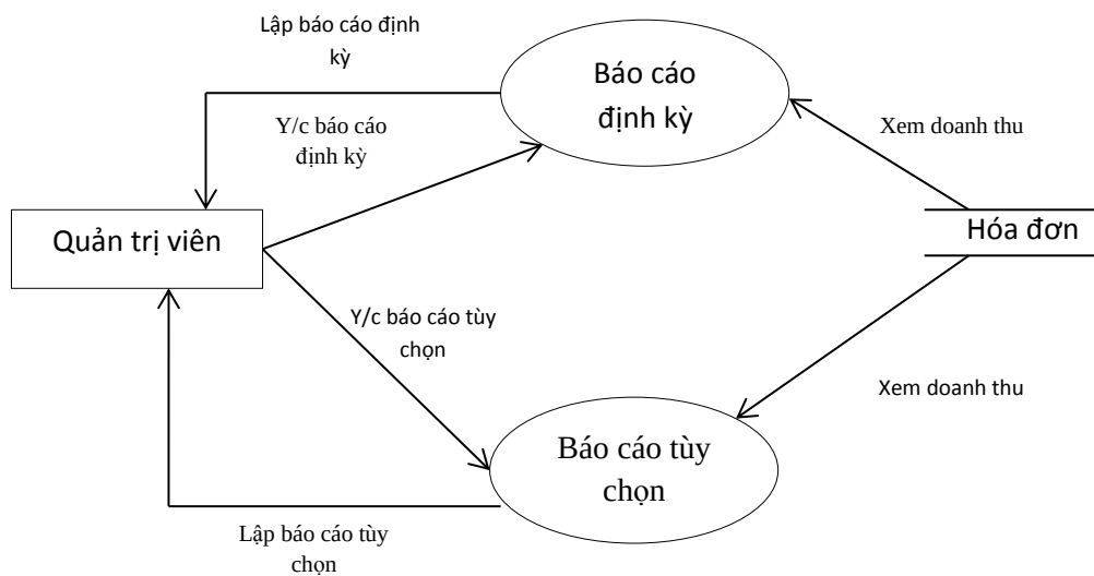
Hình 7: Mức 1- Tiến trình báo cáo
