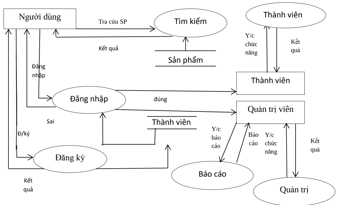
Hình 4: Biểu đồ luồng dữ liệu mức đỉnh
