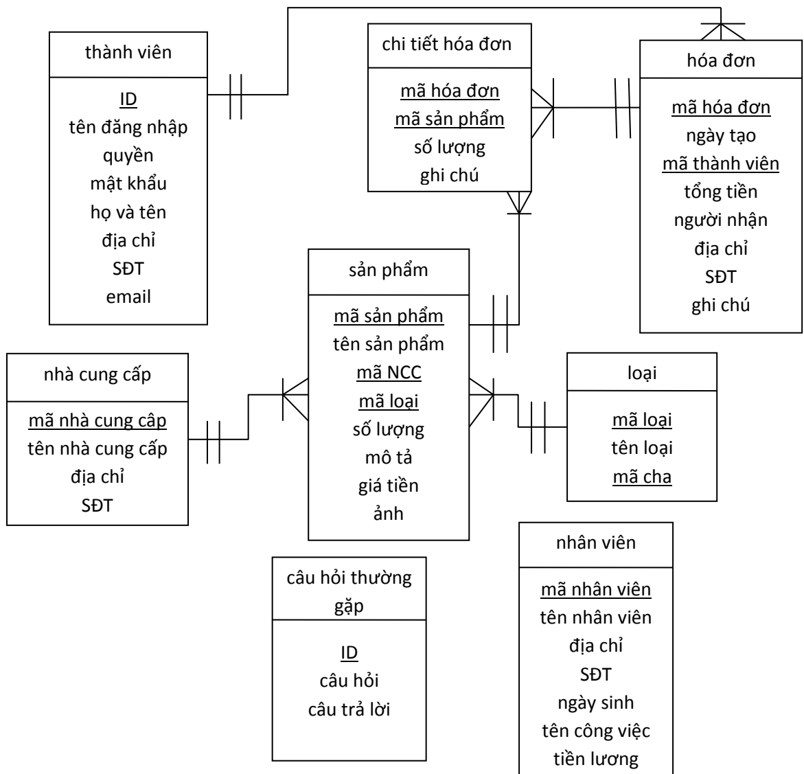
Hình 10: Biểu đồ liên kết quan hệ
