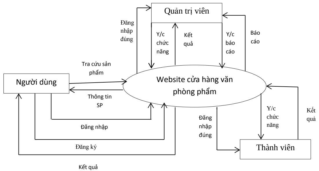
Hình 3: Biểu đồ luồng dữ liệu mức ngữ cảnh
