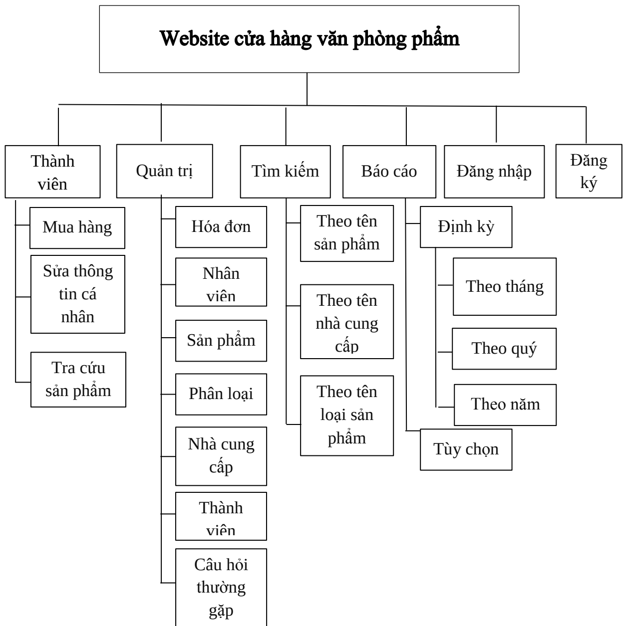
Hình 2: Biểu đồ phân rã chức năng
