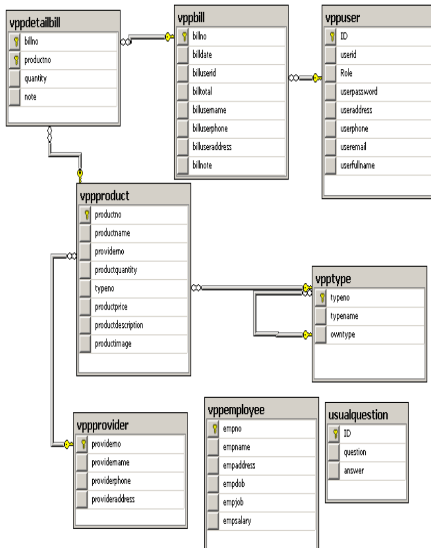
Hình 11: Sơ đồ quan hệ cơ sở dữ liệu
